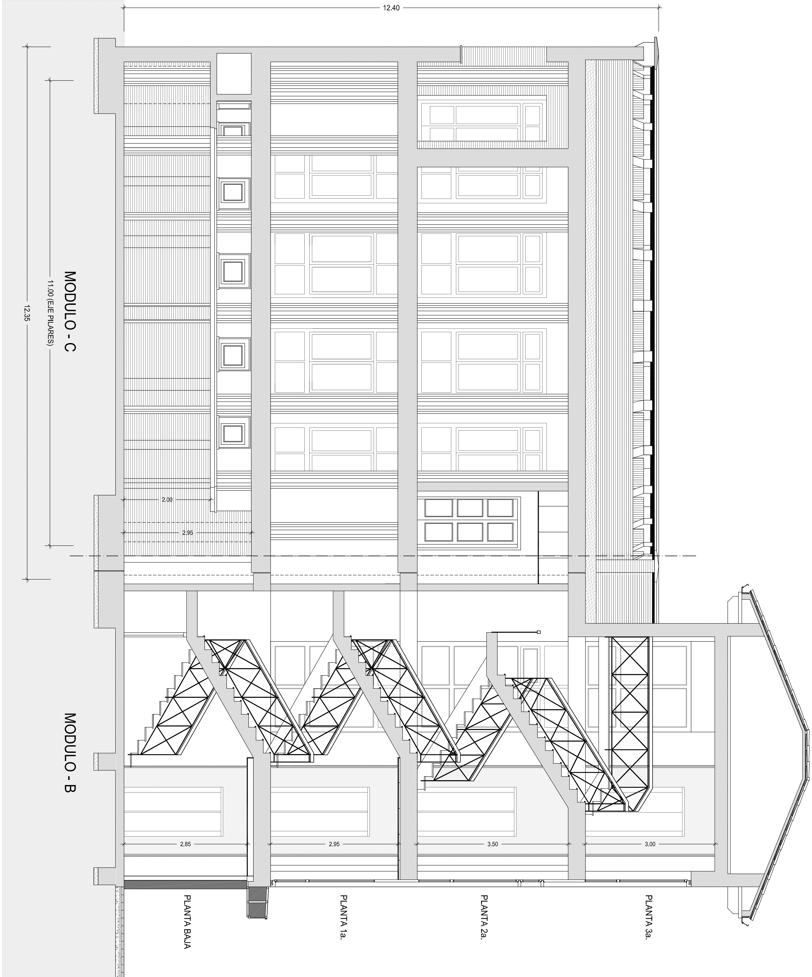
SECCION E-F
